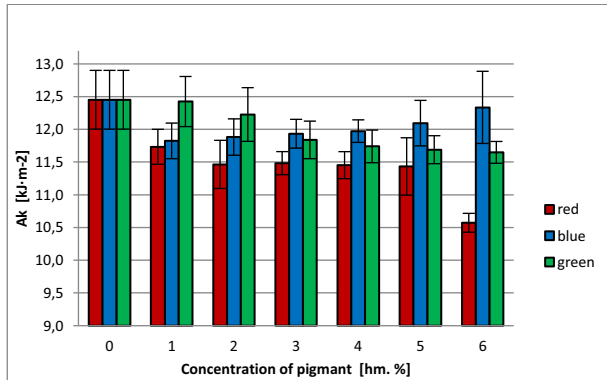
Fig 5. Noch toughness
