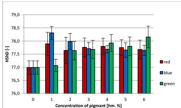
Fig 9. Shore D
